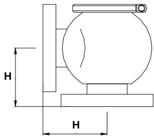
FLÄNS FLANGE
