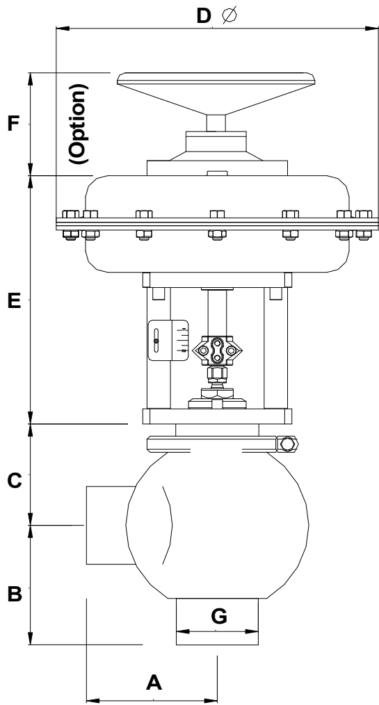
FLÄNS FLANGE
